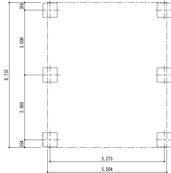
■ 基礎配置図
